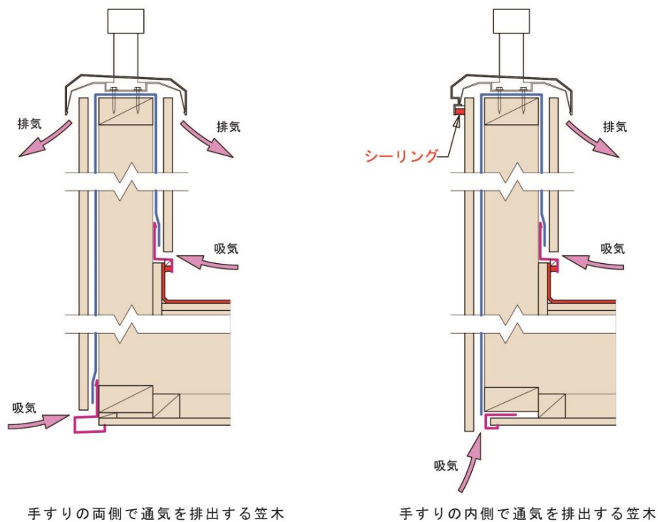
参考図8-9 手すり壁の通気構法のイメージ図
