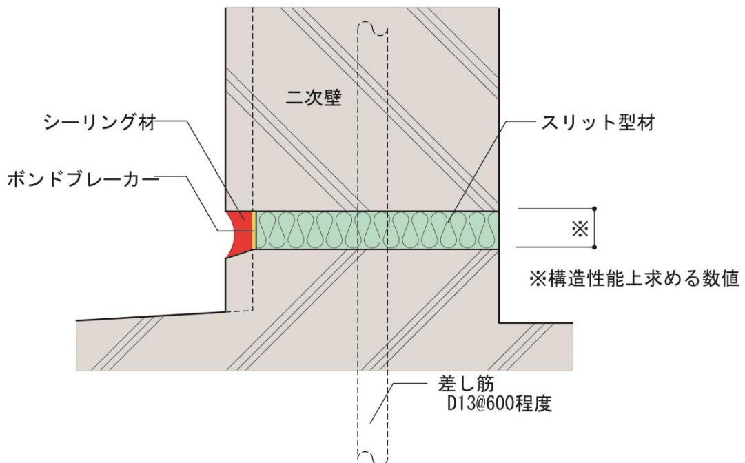
参考図21-2 耐震スリット目地のシーリング例
