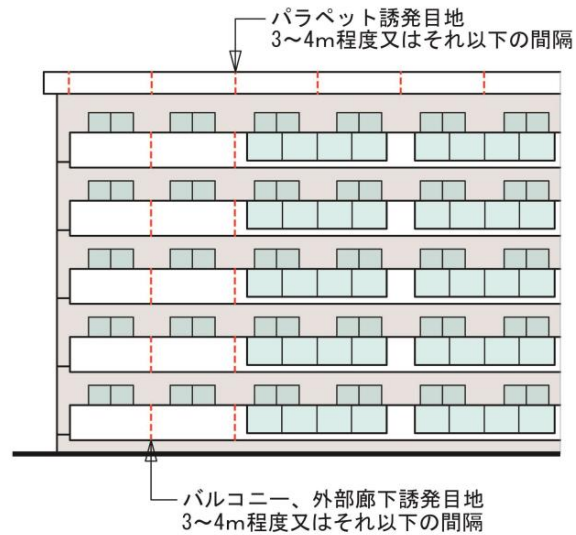
参考図21-4 ひび割れ誘発目地の設置例
