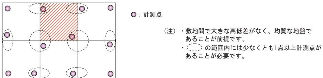
参考図4-1 隣地の計測点を含めて4点とみなすことができる例
