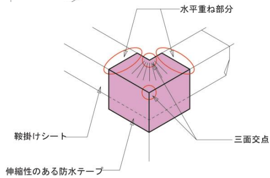
参考図8-12 手すり壁の出隅部の納まり例
