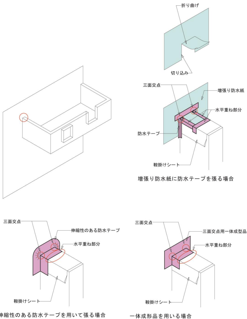
参考図8-10 手すり壁と外壁の取合い部の納まり例
